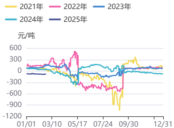
图20：焦煤5-9价差
