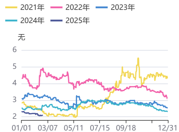
图22：焦炭/铁矿（5月）
