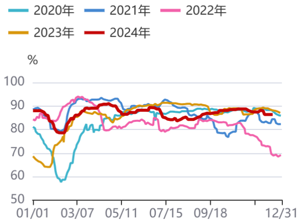
图13: 开工率: 聚酯
