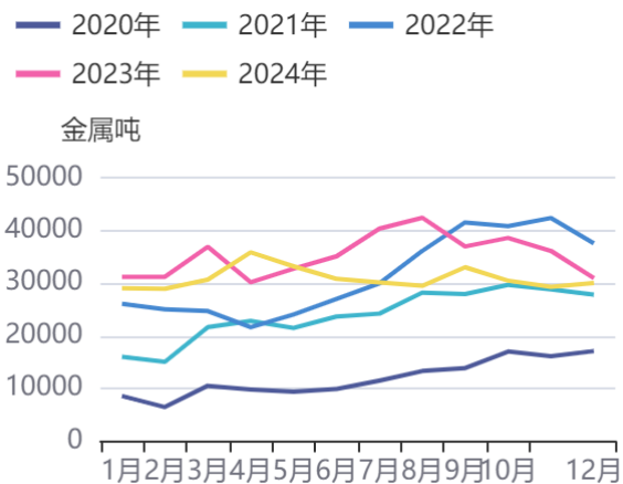
图17：硫酸镍产量
