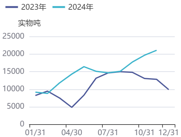
图15：六氟磷酸锂月度产量
