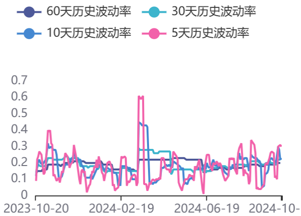
图36：历史波动率
