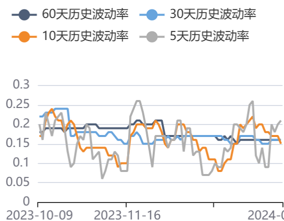
图41：历史波动率
