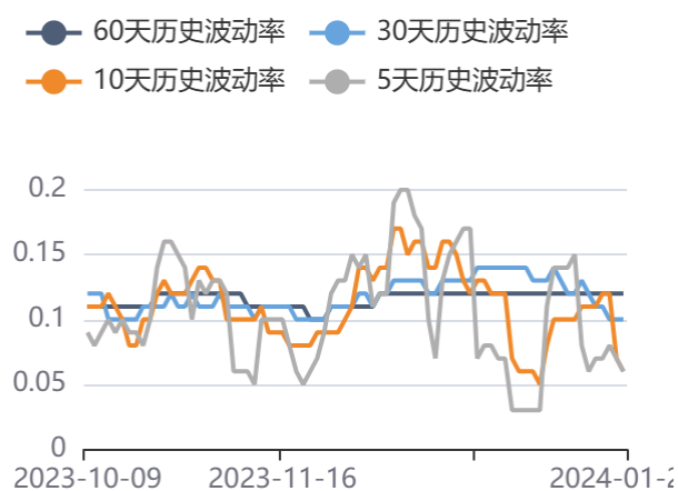
图46：历史波动率
